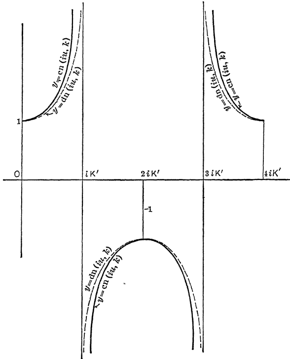
FIG. 12. y = \text{cn}(iu) ; y = \text{dn}(iu) .
